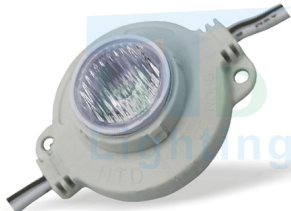
*HTD-24B 20°×60° 1.8W module
